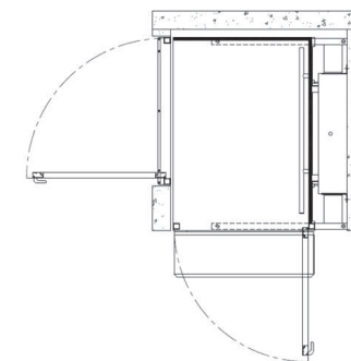
Ingresso e uscita adiacenti (90°)
