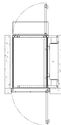
Ingresso ed uscita opposti (180°)
